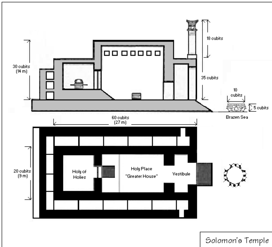
Der Salomonische Temple im Grund- und Aufriß
