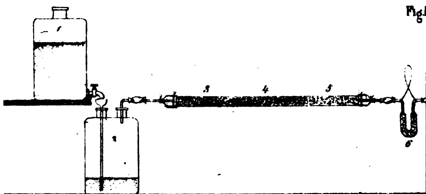
Fig. II. Apparat zur organischen Analyse
