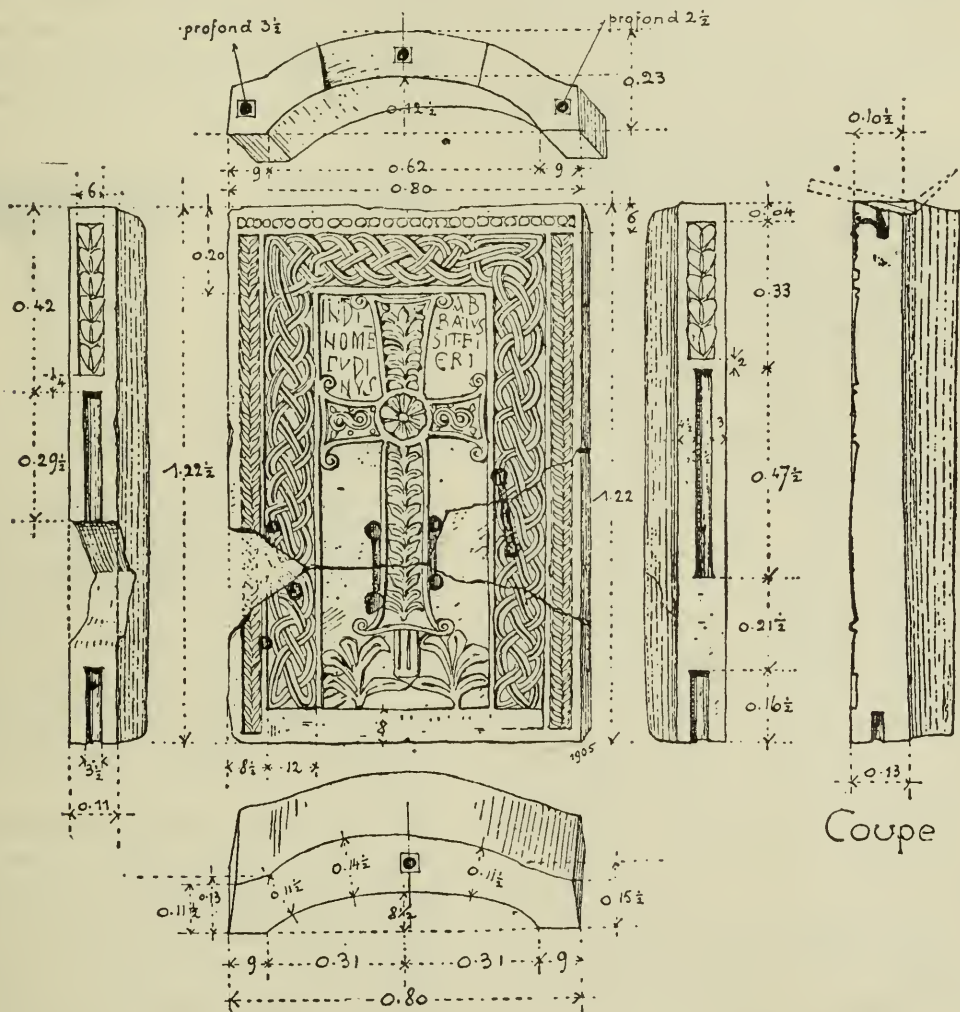
Abb. 6. Ambo von Romainmôtier. Nach Besson (A. Naef).
