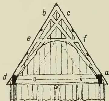
Abb. 58. Dachkonstruktion (§ 7.)
